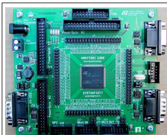
STEVAL-IFN002V1
